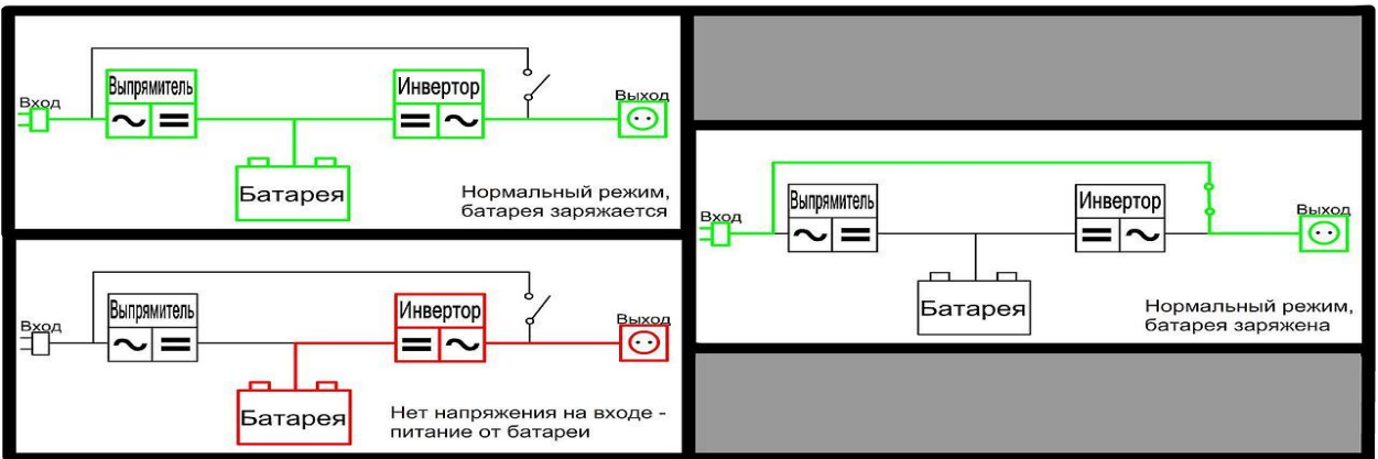
Схема работы ИБП по топологии Online
